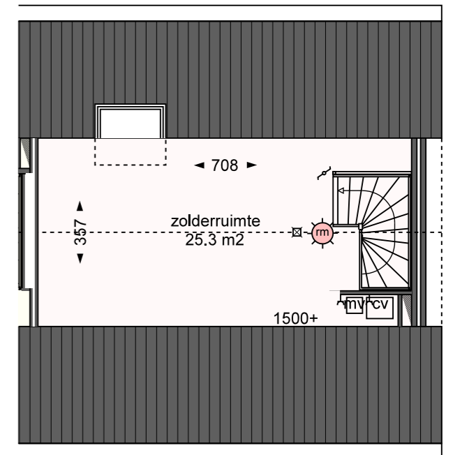
2E VERDIEPING - 25 m 2 G.O.
